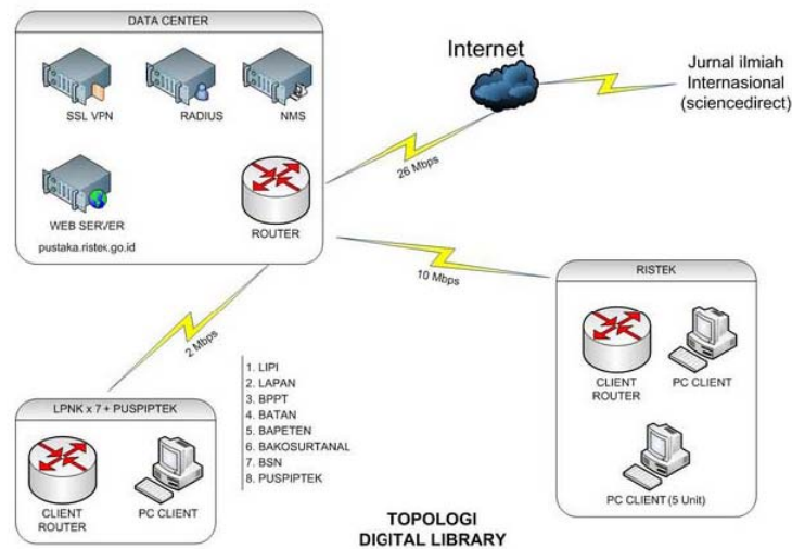
Gambar 1. Topologi jaringan digital library Pustaka Ristek (Sumber: Kemristek, 2015)
